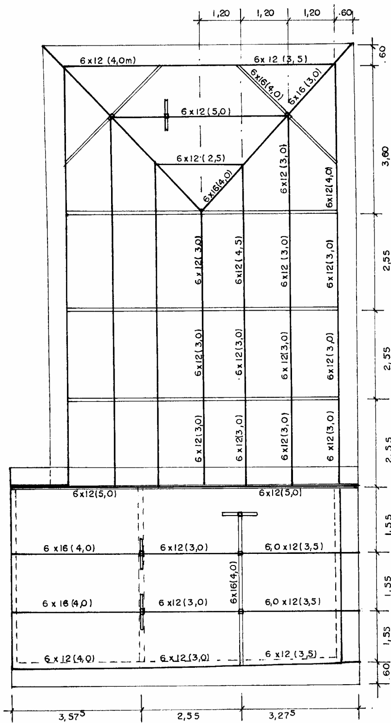
DET. ESPIGÃO
