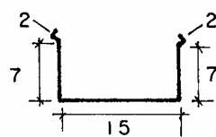
Figura 6.40 - Calha tipo coxo
