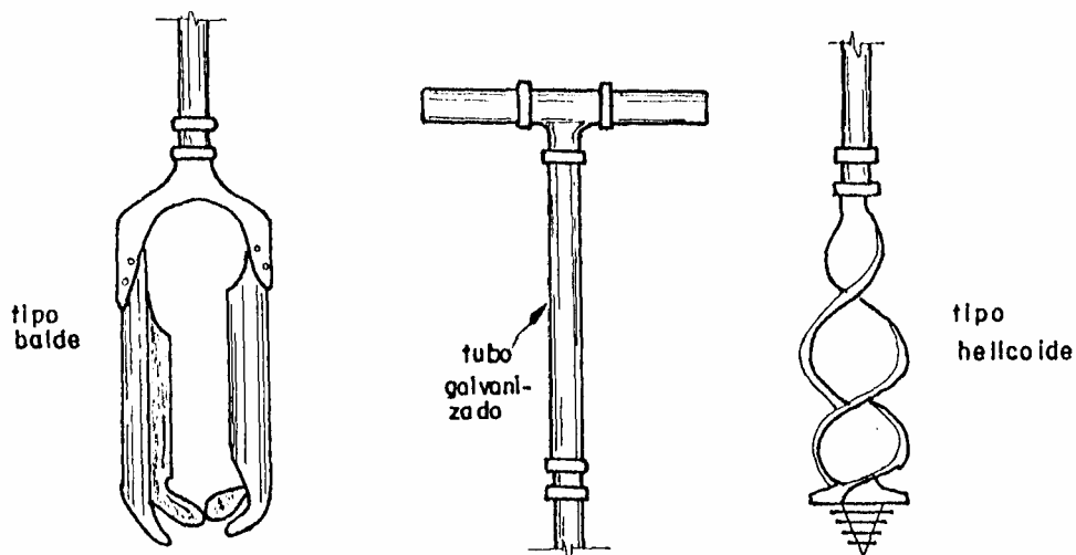
Figura 3.20 - Tipos de trado
