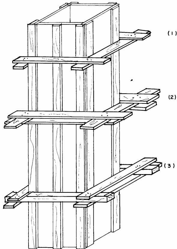
Figura 11.8 - Tipos de gravatas utilizadas em pilares (Cardão.1969)
