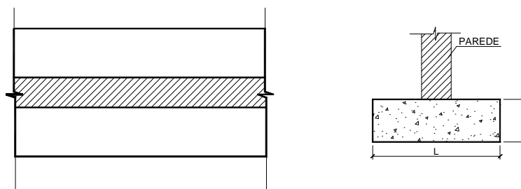
Figura 3.13 - Sapata corrida sob paredes
