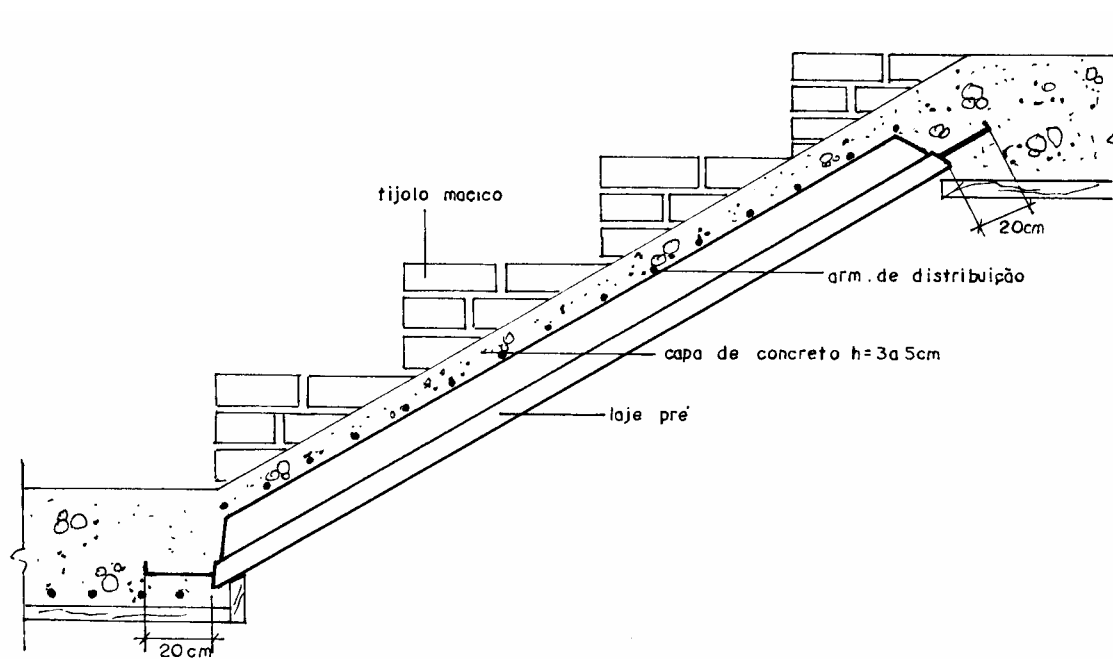
Figura 12.8 - Degraus com tijolos maciços utilizando laje pré moldada
