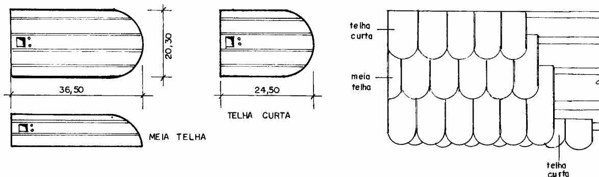
Figura 6.29- Telha Germânica
