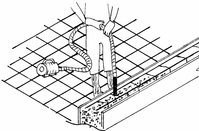
Figura 11.28 - Aplicação do vibrador na vertical
