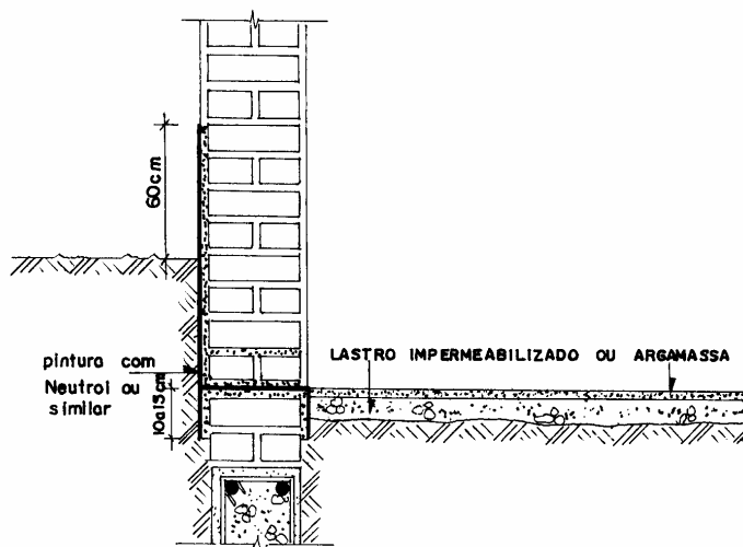
Figura 3.30 - Impermeabilização com ventilação
